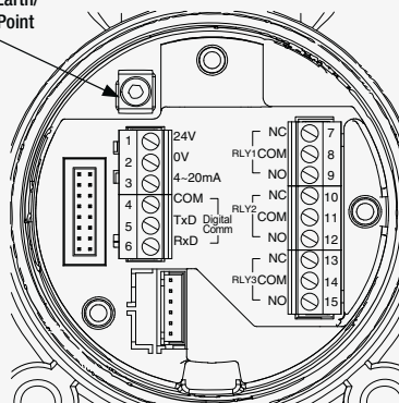
Terminal Module
