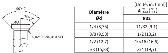
Figure 5.3 Traitement de l'évasement
