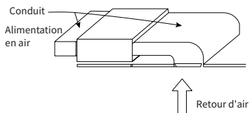
Figure 4.9 Alimentation latérale et retour arrière
