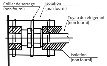
Procédure d'isolation de la tuyauterie
