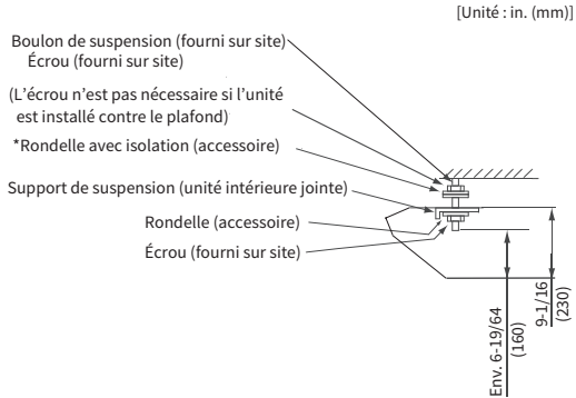
Fig.4.5 Écrous et rondelles de montage
