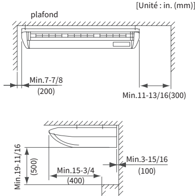
Fig.4.1 Espace pour le fonctionnement et la maintenance
