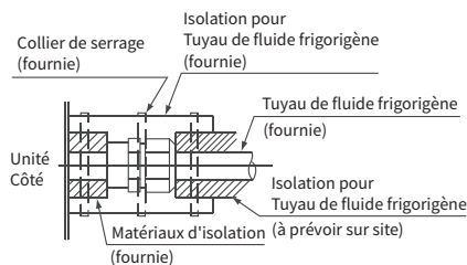
Fig.5.3 Isolation des tuyaux
