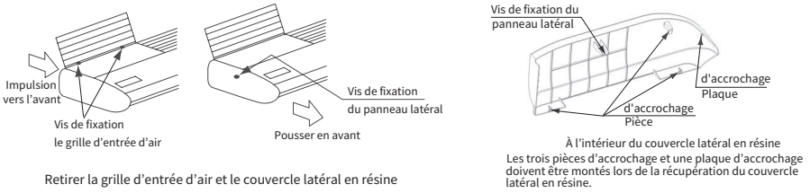
Fig.3.2 Retrait de la grille d'entrée d'air et du couvercle latéral en résine
