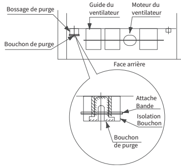
Fig.6.2 Bouchon de vidange
