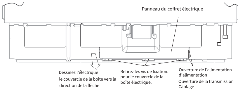
Fig.7.1 Retirer le couvercle de la boîte électrique
