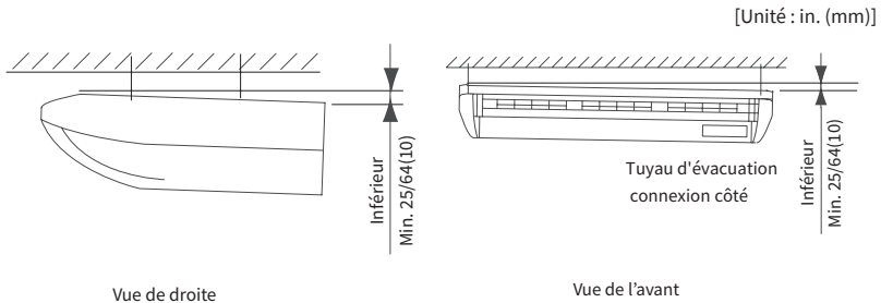
Fig.4.6 Inclinaison de l'unité de vidange pour l'installation au plafond
