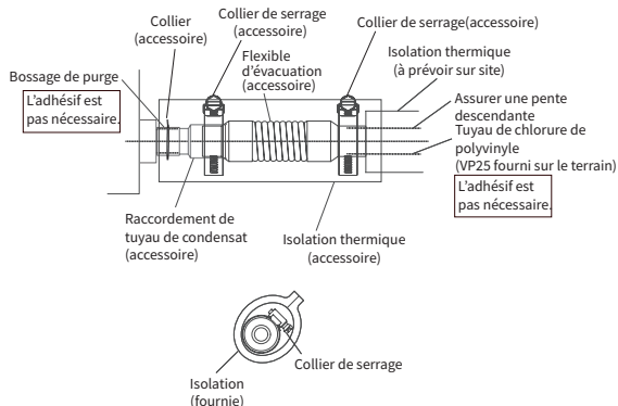
Fig.6.5 Matériau isolant d'emballage
