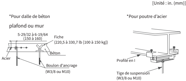
Fig.4.2 Montage des boulons de suspension
