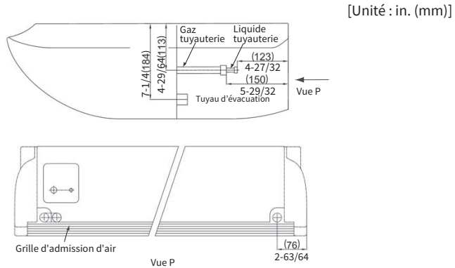
Fig.5.1 Raccordement de tuyauterie de l'unité intérieure
