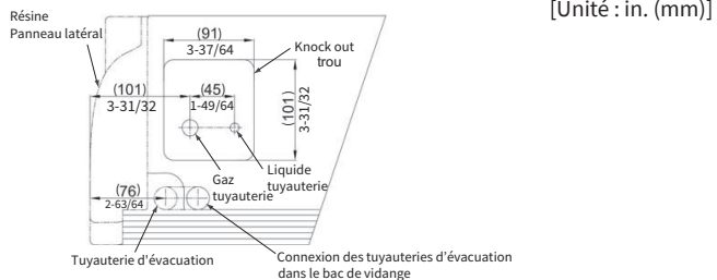
Fig.5.1 Raccordement de tuyauterie de l'unité intérieure
