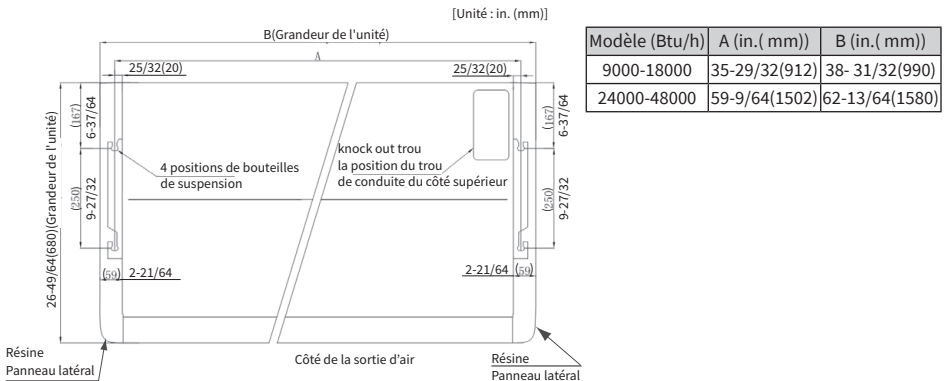
Fig.4.4 Position de montage
