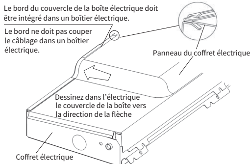
Fig.7.2 Fixer le couvercle de la boîte électrique
