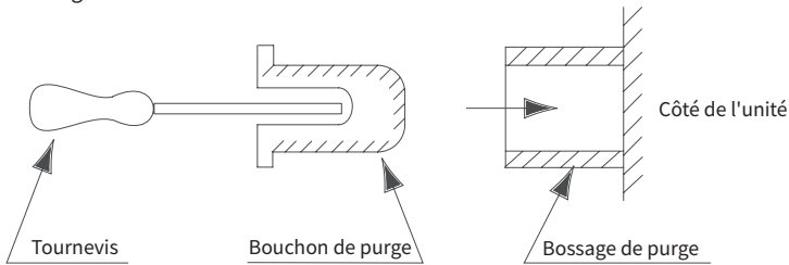
Fig.6.3 Insertion du bouchon de vidange
