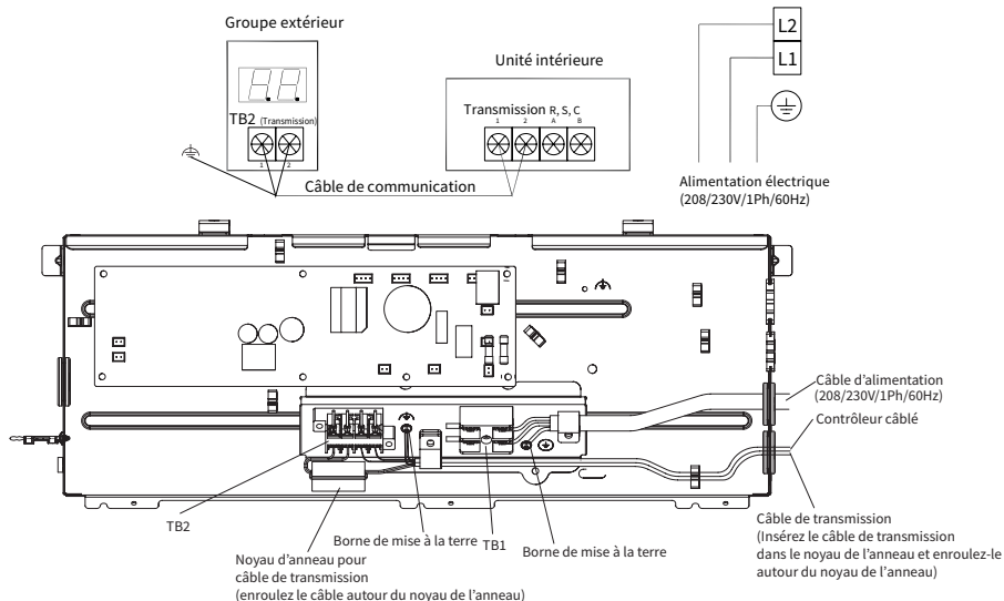
Fig.7.3 Connexion de câblage électrique pour unité intérieure
