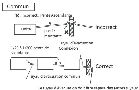
Fig.6.6 Tuyauterie de vidange
