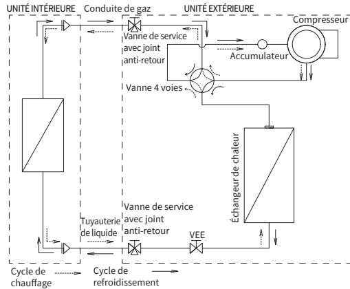
Modèle: PAS-24BLFASDQ1/PAS-30BLFASDQ1/PAS-36BLFASDQ1
