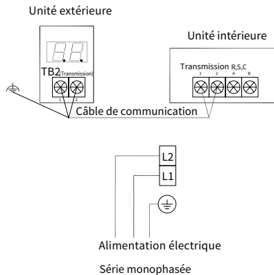
Modèle: PAS-24BLFASDQ1/PAS-30BLFASDQ1/PAS-36BLFASDQ1
